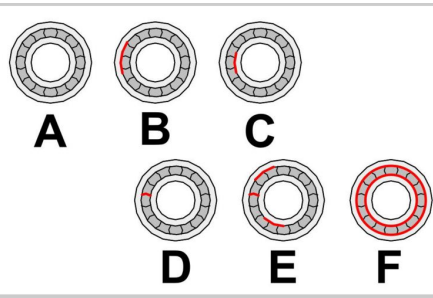
A) palier non déformé. B) palier avec déformation sur le joint torique externe. C) palier avec déformation sur le joint torique interne. D) palier avec déformation sur un corps de roulement. E) palier avec déformation sur le corps de roulement, le joint torique externe et le joint torique interne. F) palier avec forte usure.
