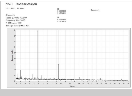
Analyse d'enveloppe d'un palier à roulement avec dommages sur le joint torique externe (B) à n=3000\text{min}^{-1}
