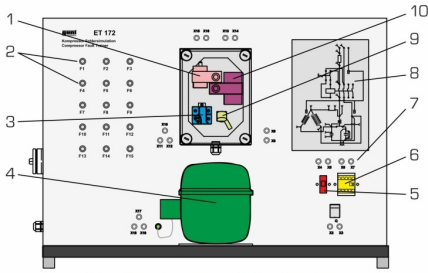
1 condensateur de service, 2 bobinopoussoirs des bornes, 3 relais de démarrage, 4 compresseur d'agent réfrigérant, 5 coupe-circuit automatique, 6 contacteur de puissance, 7 contacteurs de manoeuvre, 8 schéma de connexion, 9 protection thermique, 10 condensateur de démarrage
