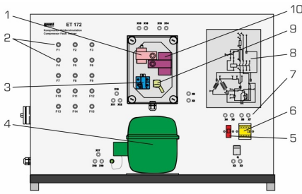
1 condensateur de service, 2 bobinopoussoirs des bornes, 3 relais de démarrage, 4 compresseur d'agent réfrigérant, 5 coupe-circuit automatique, 6 contacteur de puissance, 7 contacteurs de lecture, 8 schéma de connexion, 9 protection thermique, 10 condensateur de démarrage
